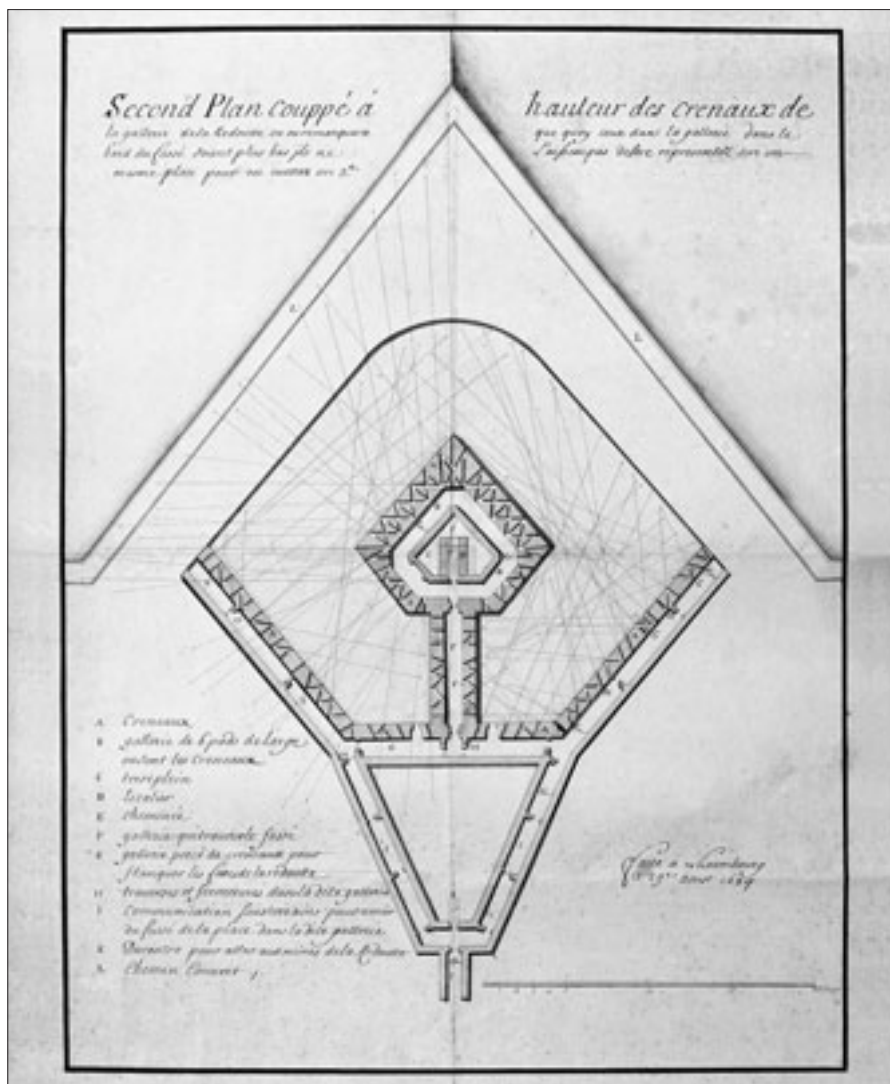
Abb. 1 Idealplan zur Errichtung eines Ravelins. Datiert 29. August 1684. 1684/85 weilte Louis de Hautebeau, ein französischer Mathematiker und Festungsingenieur, in Solothurn. Er befasste sich mit Vorschlägen zur Verstärkung der Schanzenanlage um die Altstadt. In seinem vom 2. Dezember 1684 datierten Gutachten betont er mehrmals die Notwendigkeit, den Schanzengraben auszuweiten und Ravelins (Vorschanzen) hineinzubauen. (Quellenhinweis: Ratsmanual 189/1685/37 und Schanzschriften.)
