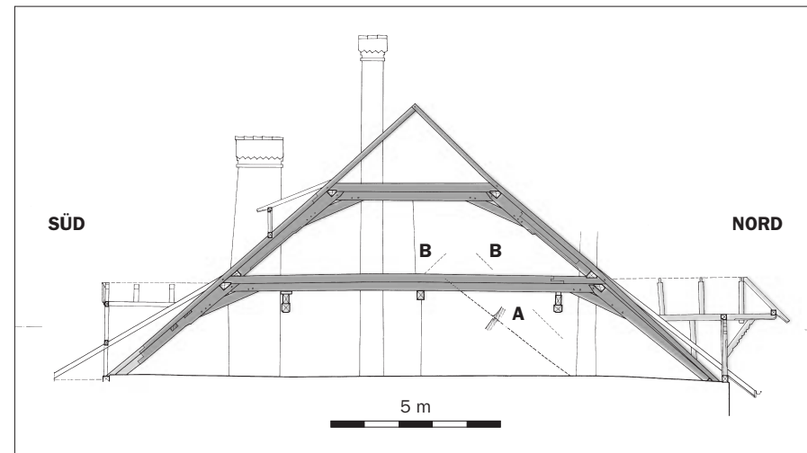
Abb. 9 Querschnitt durch die Dachkonstruktion, Blick nach Westen an die Brandmauer. Mittelgrau gerastert: Konstruktionsteile von 1596/97. Hellgrau gerastert: Konstruktionsteile von 1714/15. A ältere Dachlinie, Phase A, 15. Jahrhundert. B ältere Dachlinie Nachbarhaus West. Weiss: Konstruktionsteile 18./19. Jahrhundert.
