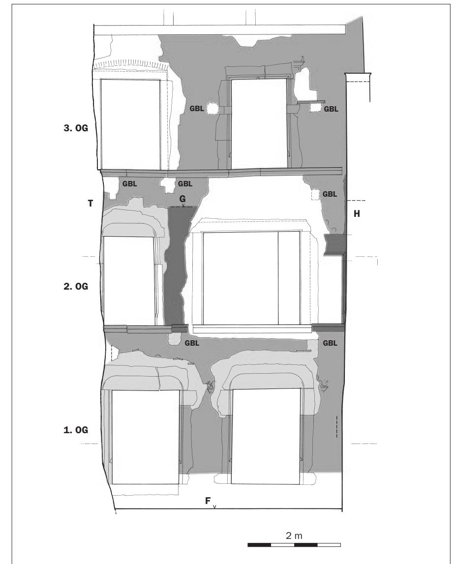
Abb. 3 Hoffassade Vorderhaus, Planaufnahme nach den baugeschichtlichen Sondierungen und dem Entfernen defekter Verputzpartien. Dunkelgrau gerastert: Mauerwerk Phase 1, 15. Jahrhundert mit Rest eines dazugehörigen Fenstergewändes in situ. G Grenze im Mauerwerk. H Hofmauer, ältere Höhe. Mittelgrau gerastert: Verputz (1. OG) bzw. Mauerwerk mit Verputz (2., 3. OG) Phase 2, 16. Jahrhundert. T Treppenturm mit nachträglich zurückgearbeiteter Front, älteste Teile Phase 2. Hellgrau gerastert: Verputz/Mauerwerk Phase 3, 17. Jahrhundert. Weiss: Verputz/Mauerwerk Phase 5, 6, 18./19. Jahrhundert. F Flachdach von 1983. Das Hofniveau lag bis dahin um ein Geschoss tiefer. GBL Gerüstbalkenlöcher aus verschiedenen Phasen.
