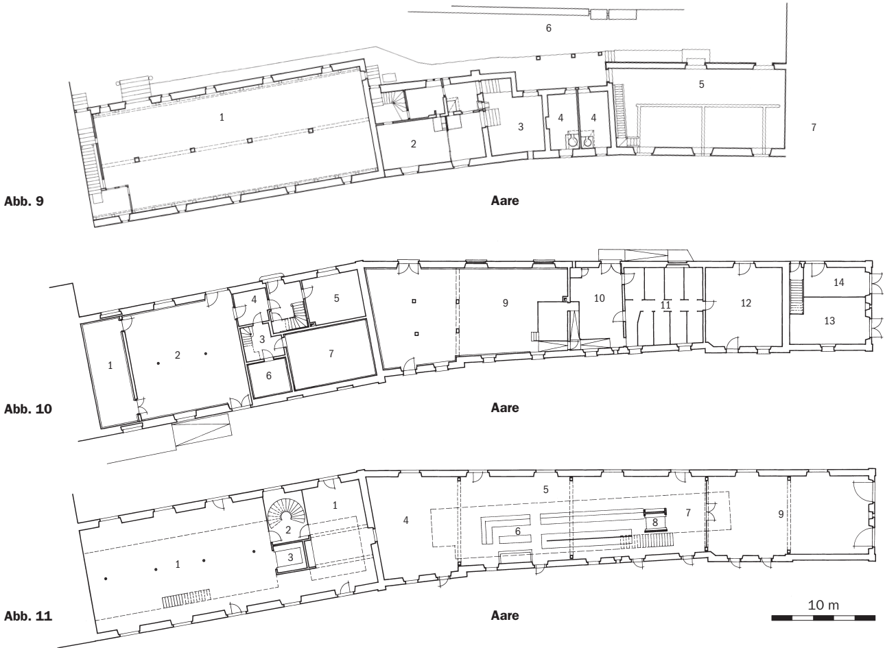
Abb. 11 Grundriss, Zustand nach dem Umbau von 2001/2002. Raumfunktionen: 1 Ausstellung/Verkaufslokal; 2 Treppenhaus; 3 Lift; 4 Restaurant; 5 Bar; 6 Küche; 7 Foyer; 8 Lift; 9 Kulturraum. Gestrichelt eingezeichnet neues Zwischenpodest über 1 bzw. Neben- raum-Kubus über 5, 6, 7.
