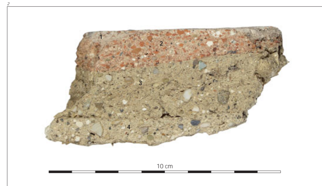
Abb. 2 Aufbau und Zusammensetzung der Mörtel- und Verputzschichten: 1 Weisse Malschicht aus Kalk mit Quarz- und Ziegelsplitt; 2 Ausgleichs- und Isolationschicht aus rosarotem Kalkmörtel mit Ziegelsplitt; 3 Zwischenschicht aus Kalkmörtel mit beige Sand und etwas Kies; 4 Mauerputzschicht oder Zwischenschicht aus Kalkmörtel mit weiss-beigem Sand und etwas Kies.
