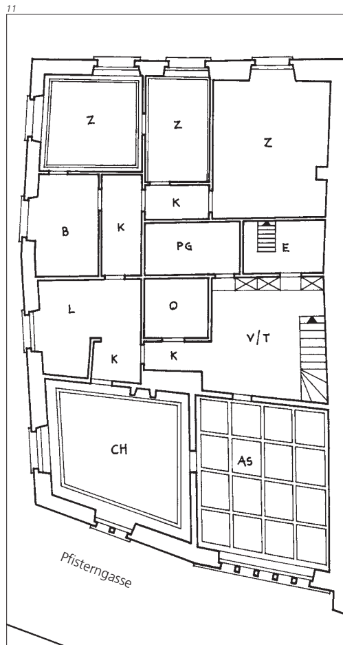
Abb. 12 Grundriss 1. Obergeschoss, im heutigen Zustand, nach dem Umbau von 2006.
