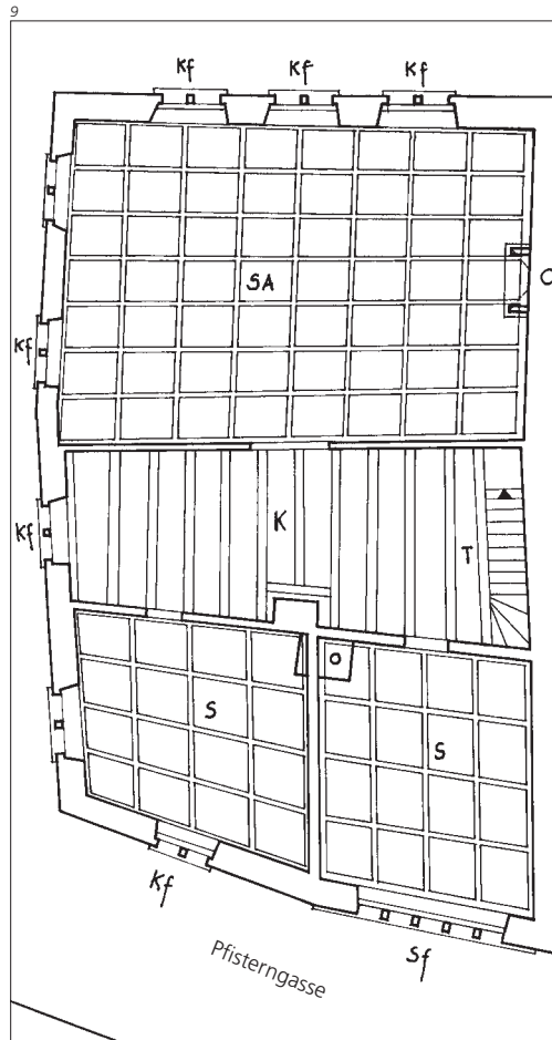
Abb. 9 Grundriss 1. Obergeschoss, Rekonstruktion Zustand um 1650 nach der baulichen Zusammenfassung der zwei bisher selbständigen Häuser. Der Grundriss, der herrschaft- lichen Ansprüchen angepasst ist, enthält im Norden einen grossen Festsaal, der durch einen breiten Korridor von den beiden nach Süden orientierten Stuben getrennt ist.
