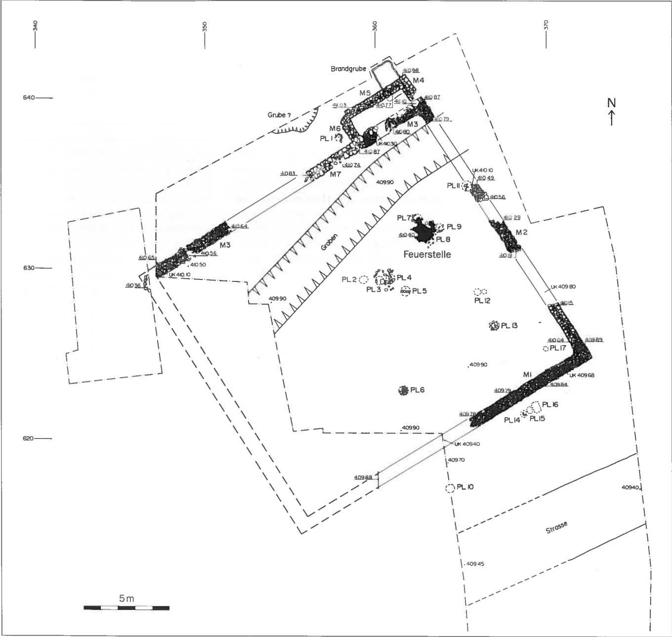
Abb. 34 Olten/Feigelfhof, Solothurnerstrasse 116. Gesamtplan des Gebäudes.
