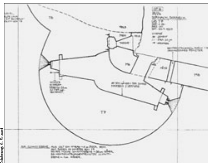
Abb. 24 Dornach, Ruine Dorneck. Grundriss der Nordwestecke (M6/M6N) des Nordwestbaus und des westlichen Zwillingsturmes (T7), 1. Geschoss, Mst. 1:150.
