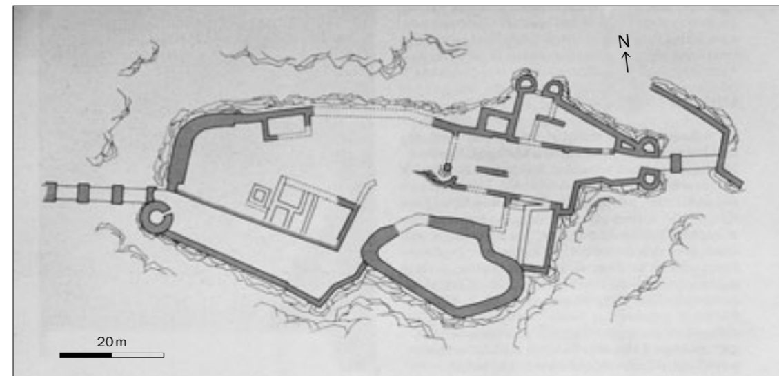
Abb. 17 Pfeffingen (BL), Ruine Pfeffingen. Grundriss, Mst. 1:1000. Aus: Meyer 1981/1, S. 114.
