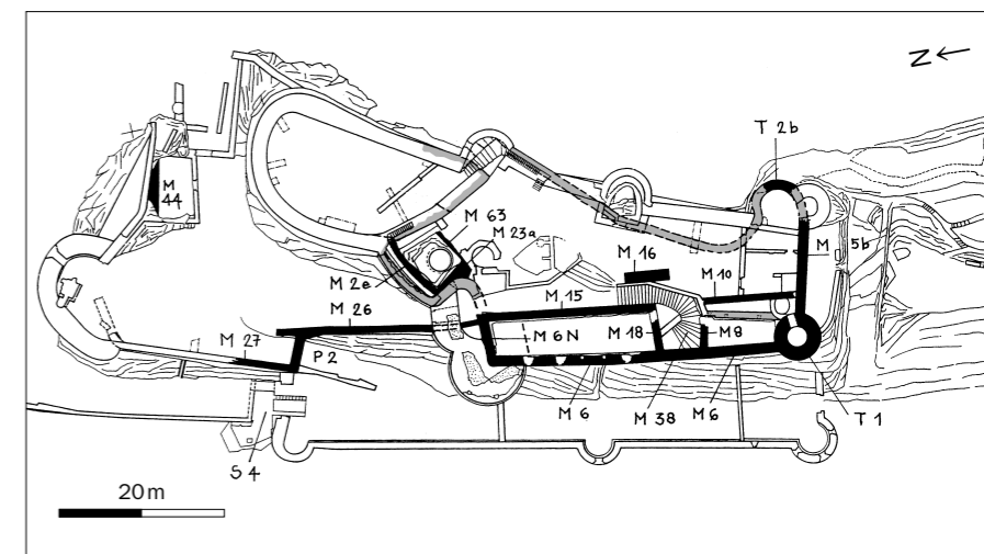
Abb. 21 Dornach, Ruine Dorneck. Bauphase III, Mst. 1:1000. Schwarz: Neubau/Umbau. Gerastert: aus der vorhergehenden Bauphase übernommenes Mauerwerk. Gestrichelt: Rekonstruktion. Der Hexenturm (T1) ist auf der Höhe des obersten Geschosses, der Nordwestbau (M6, M6N, M15, M18) auf der Höhe des zweiten Geschosses geschnitten.
