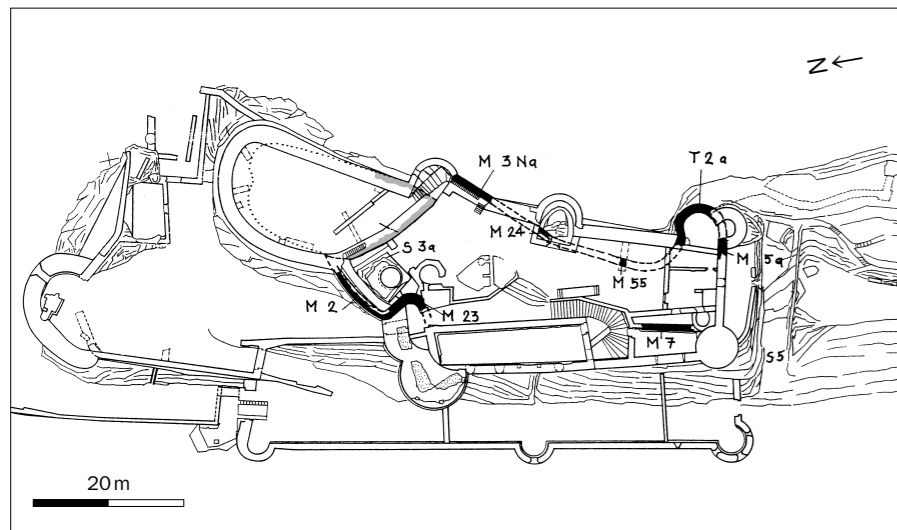
Abb. 19 Dornach, Ruine Dorneck. Bauphase II, Mst. 1:1000. Schwarz: Neubauten. Gerastert: aus der vorhergehenden Bauphase übernommenes Mauerwerk. Gestrichelt: Rekonstruktion.
