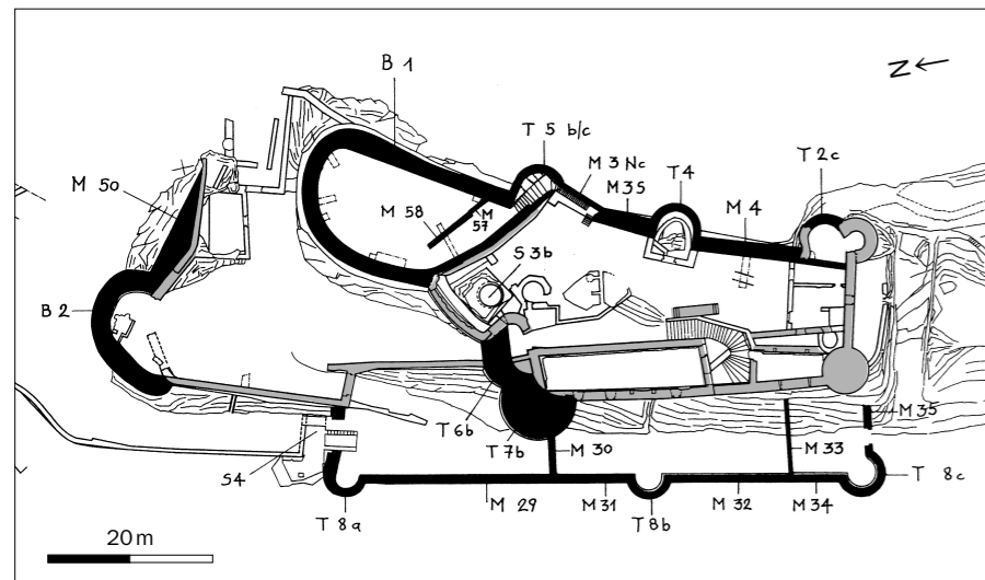
Abb. 42 Dornach, Ruine Dorneck. Bauphase VI, Mst. 1:1000. Legende vgl. Abb. 21.
