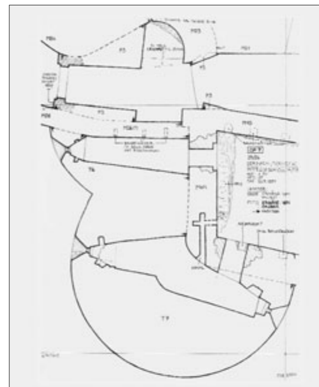
Abb. 39 Dornach, Ruine Dorneck. Zwillingstürme (T6/T7) und oberes Tor (P3), Grundriss des ersten (T6/P3) respektive zweiten (T7) Geschosses, Mst. 1:150.
