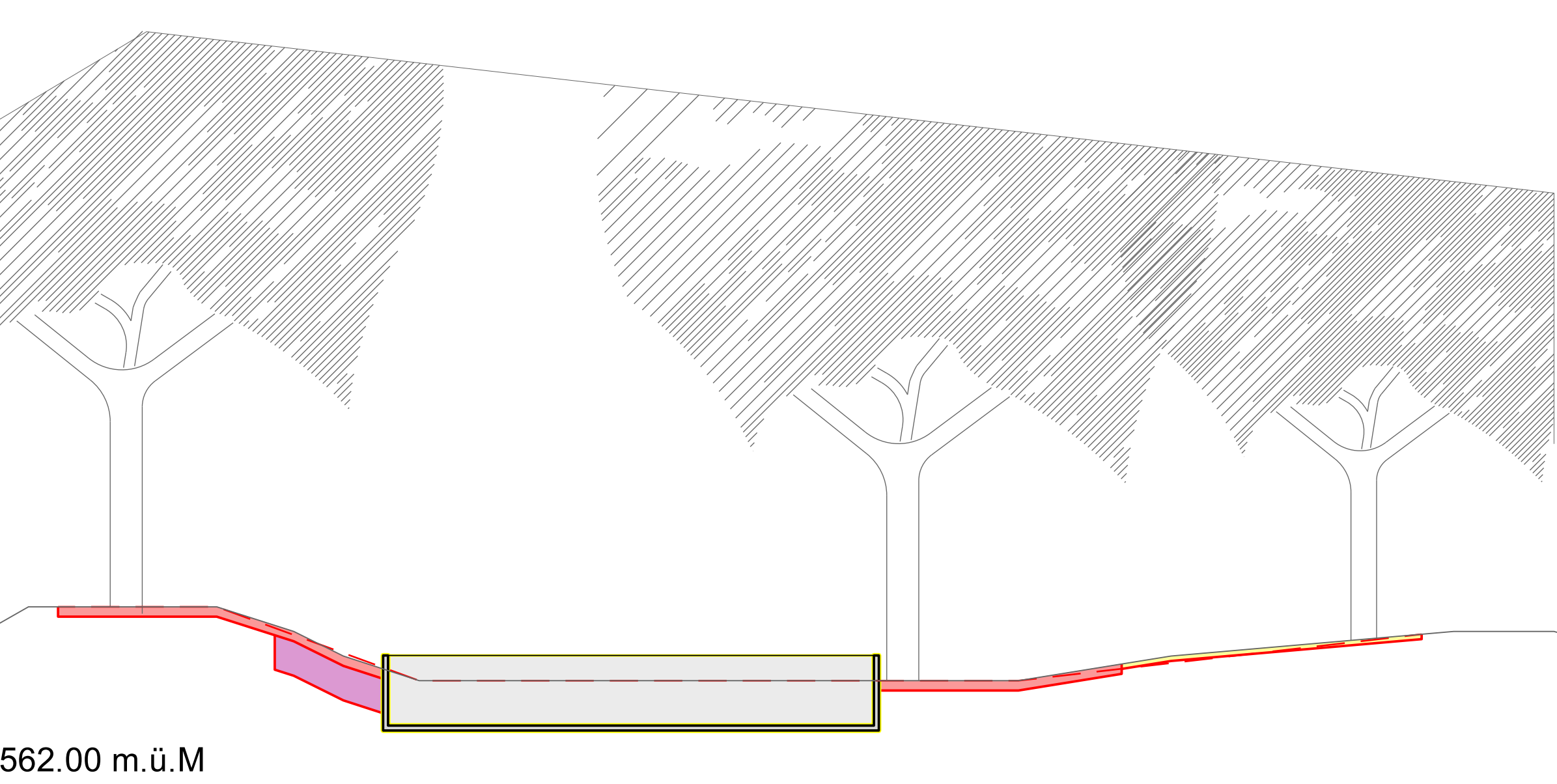
Schnitt B - B , 1 : 200
