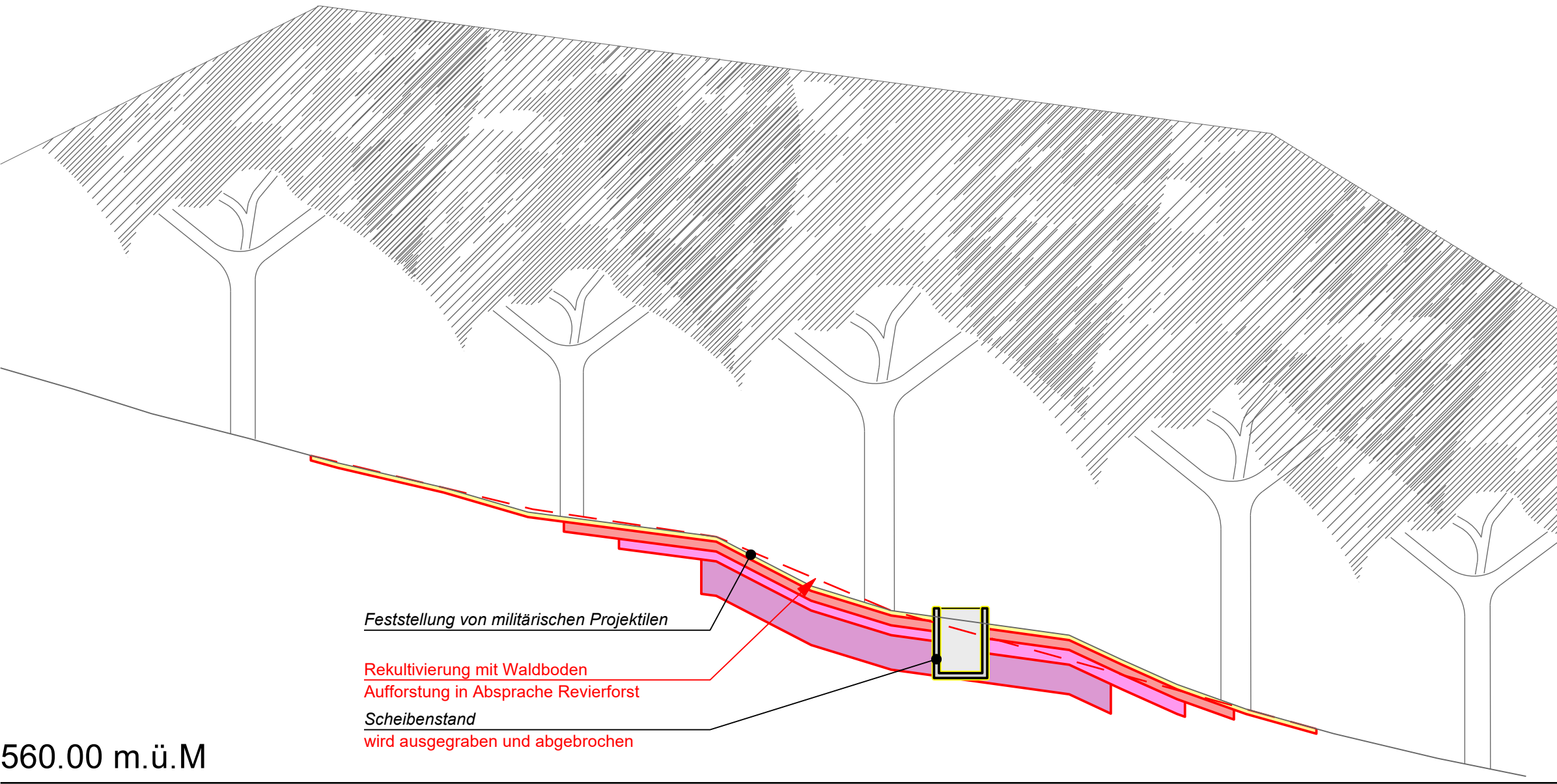
Schnitt A - A, 1 : 200
