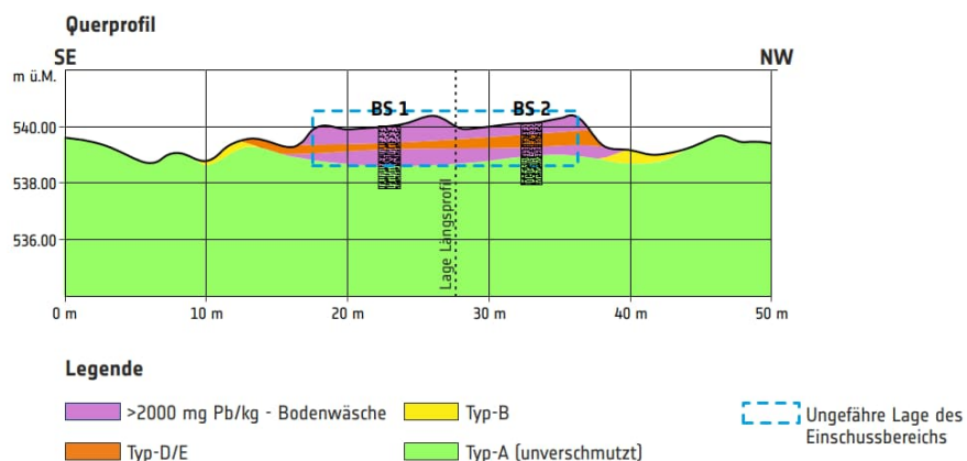
Abb. 3: Querprofil durch den Aushubbereich gemäss vorgängiger Schadstoffuntersuchung, Quelle: Bericht Vor- und Sanierungsuntersuchungen, magma ag, 2021.
