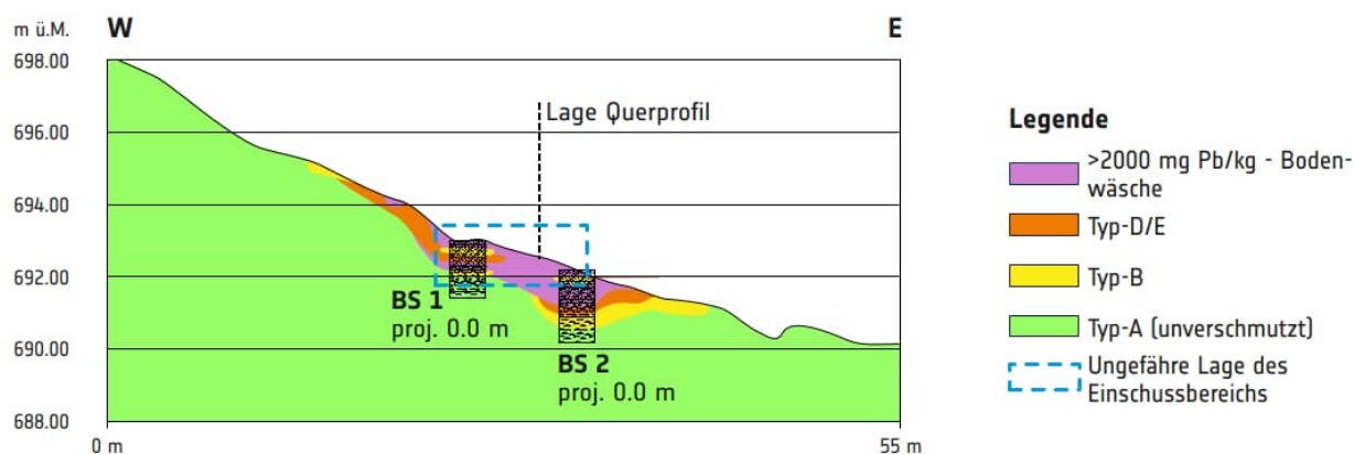
Abb. 3: Querprofil durch den Aushubbereich gemäss vorgängiger Schadstoffuntersuchung, Quelle: Bericht Vor- und Sanierungsuntersuchungen, magma ag, 2021.
