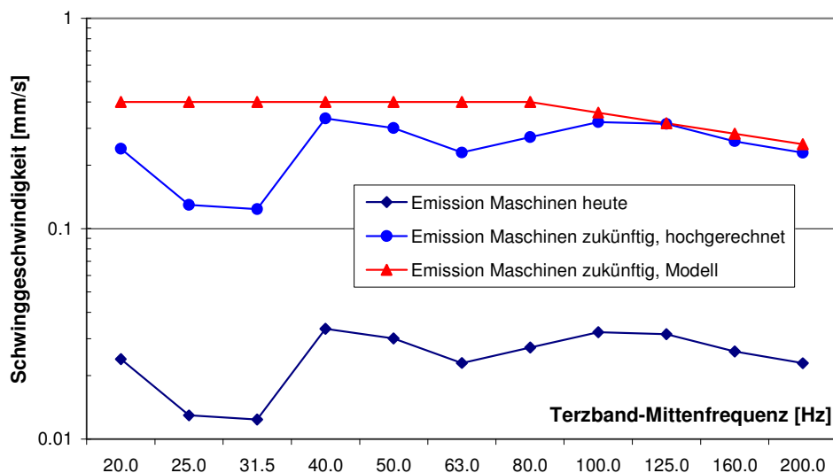
Abb. 2: Emissionsspektren der Turbinen heute zukünftig (Prognose).
