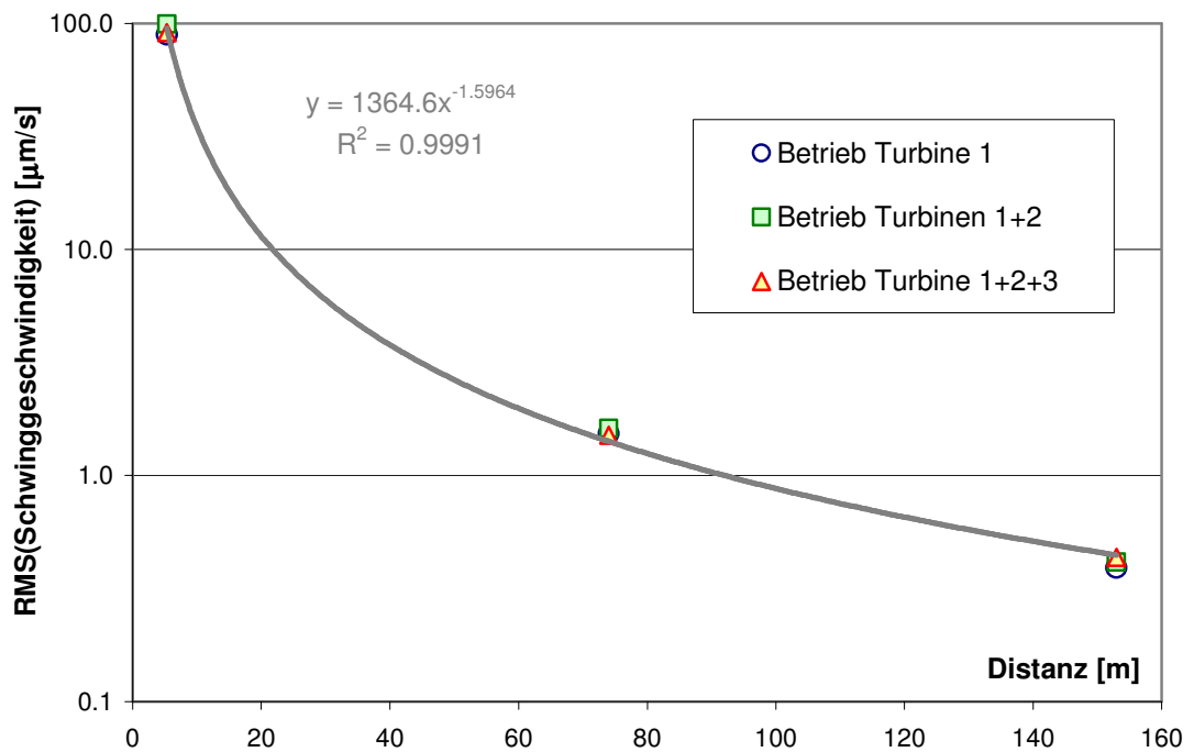
Abb. 4: Abstandsabnahme der Schwinggeschwindigkeiten infolge Maschinenbetrieb.
