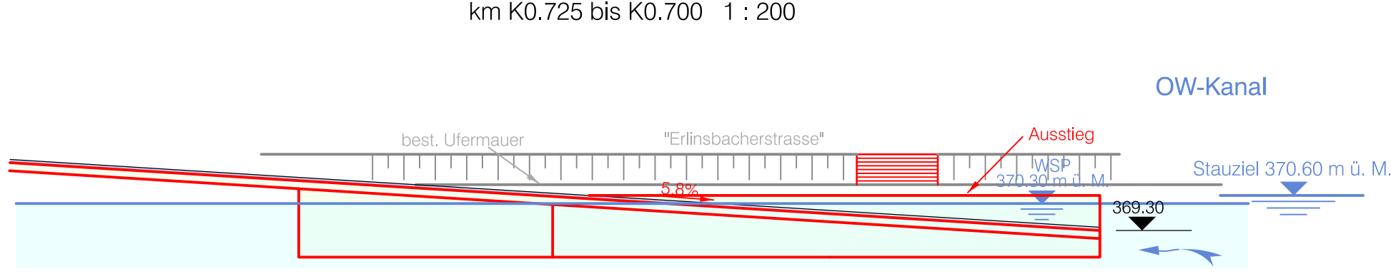
Ansicht D - D km K0.725 bis K0.700 1 : 200
