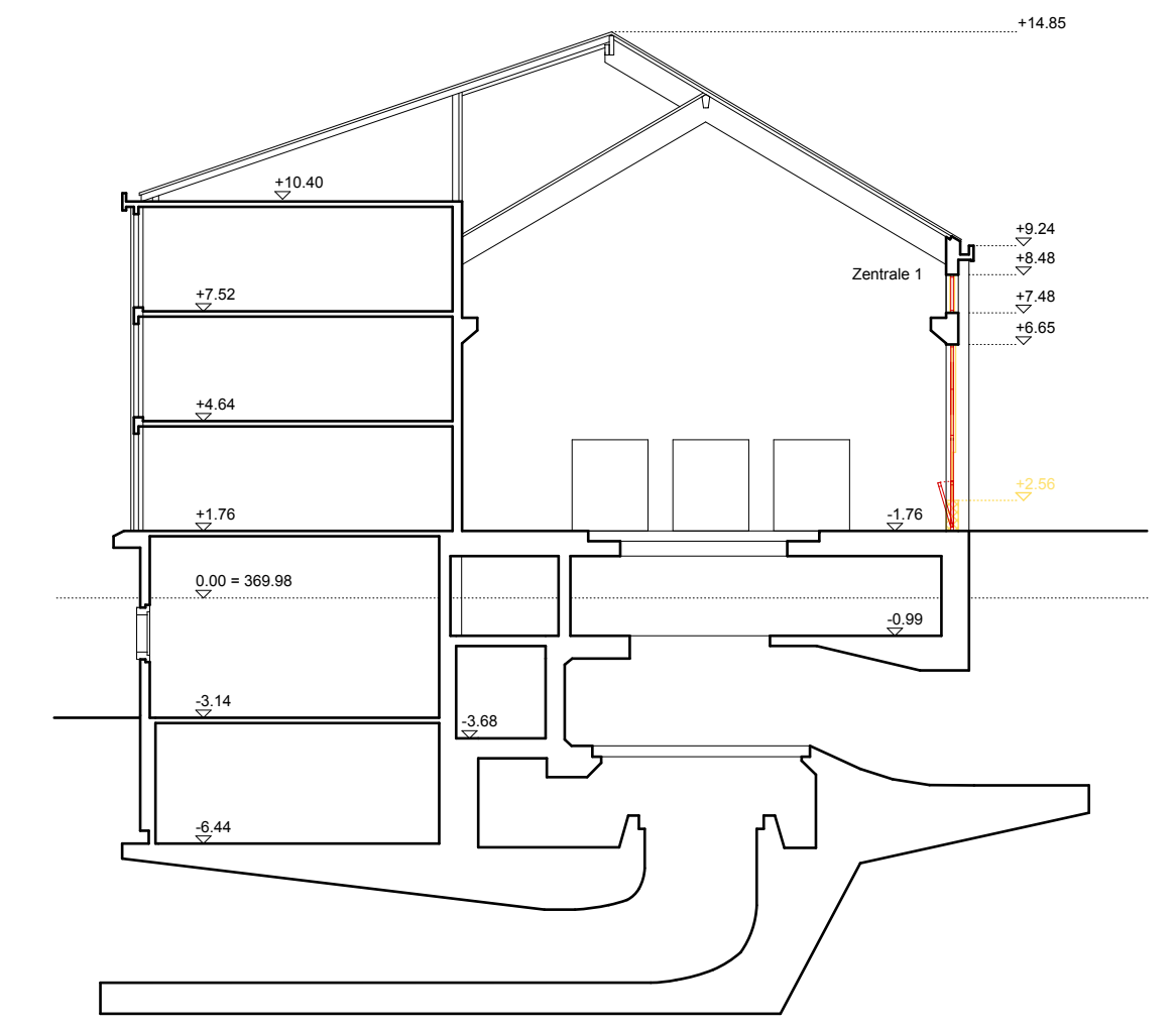
Schnitt E-E
