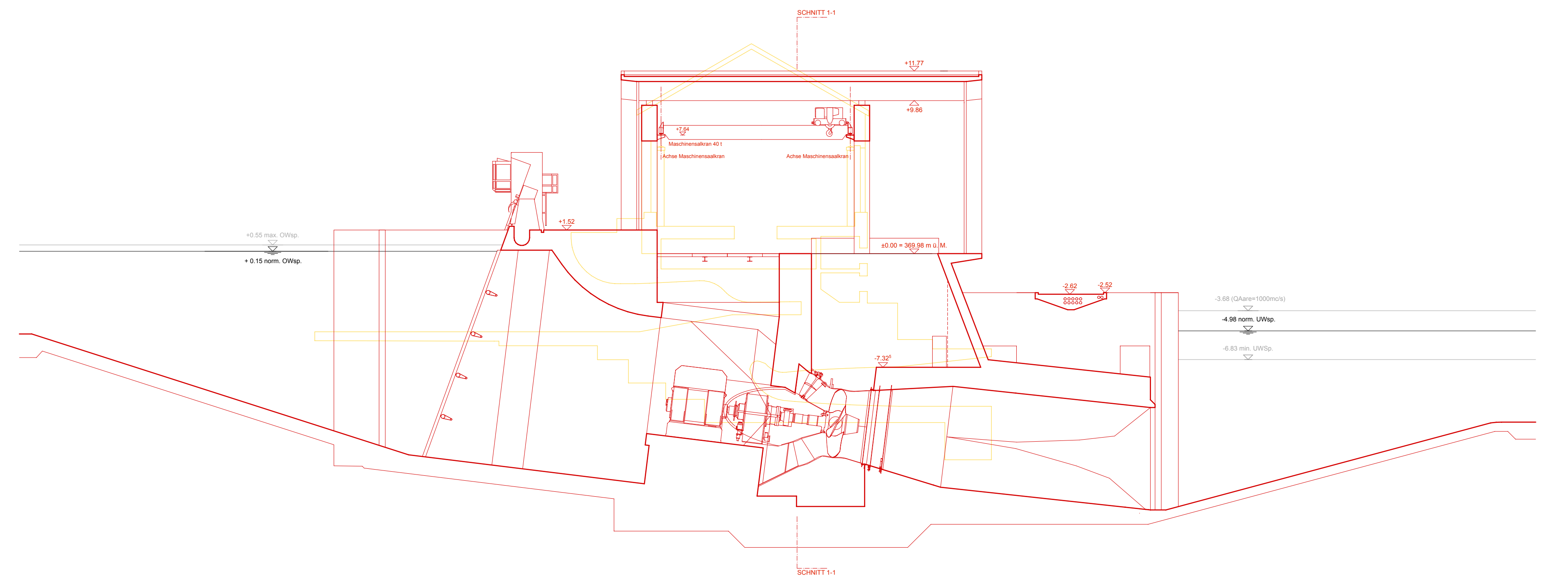
Schnitt C-C
