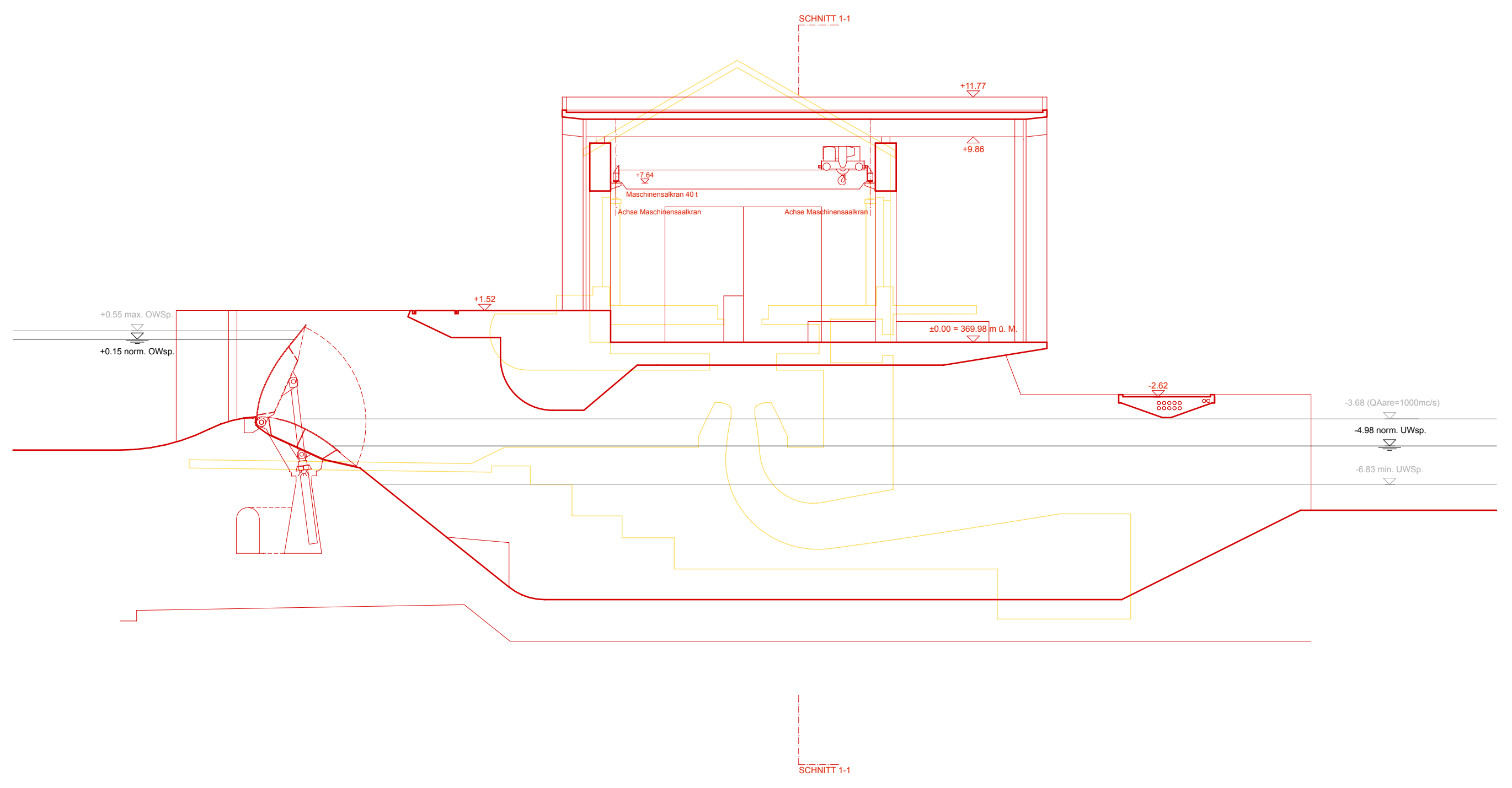
Schnitt B-B
