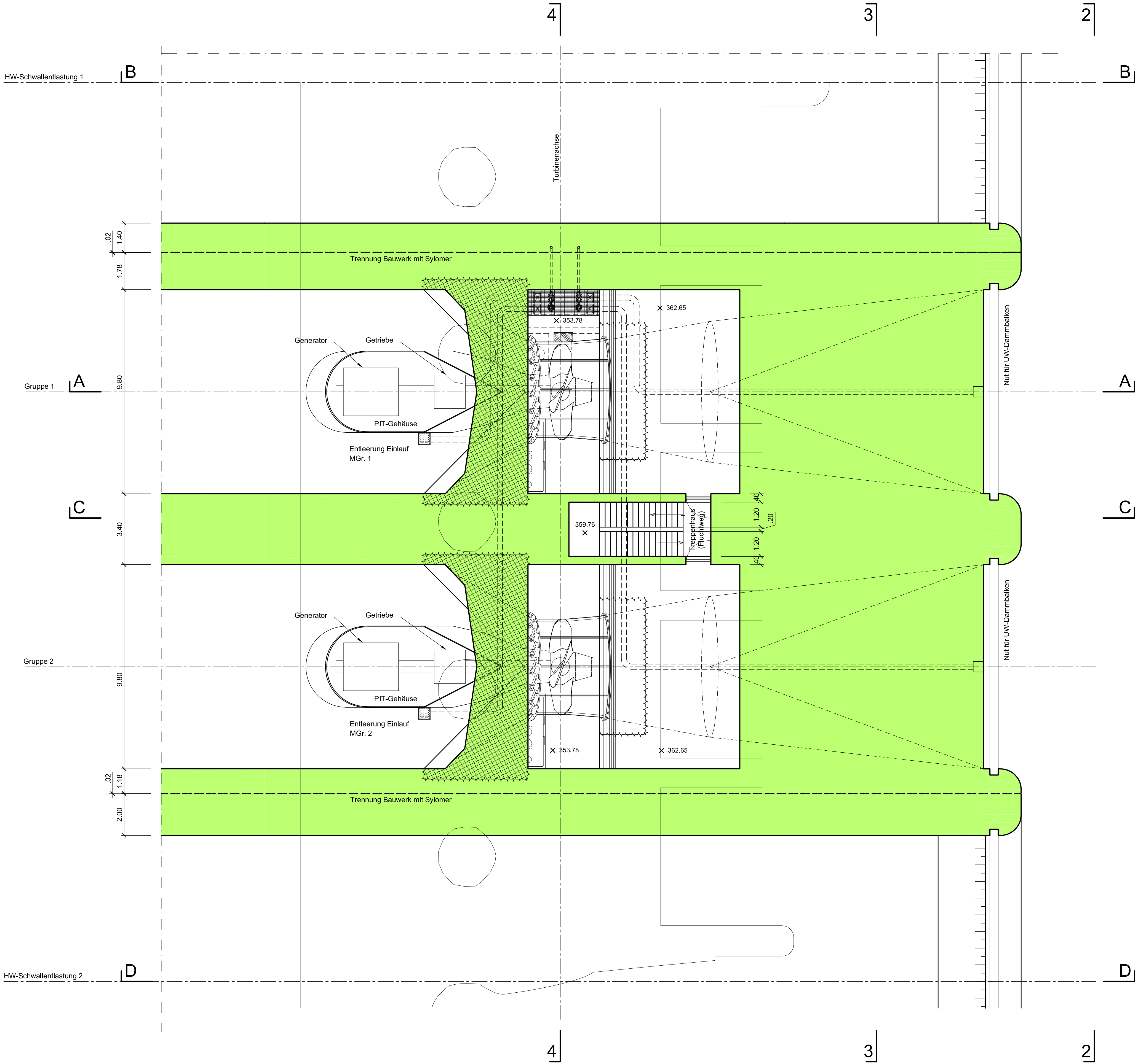
Grundriss auf Ebene Saugrohrdecke 1:100 Kote 362.65
