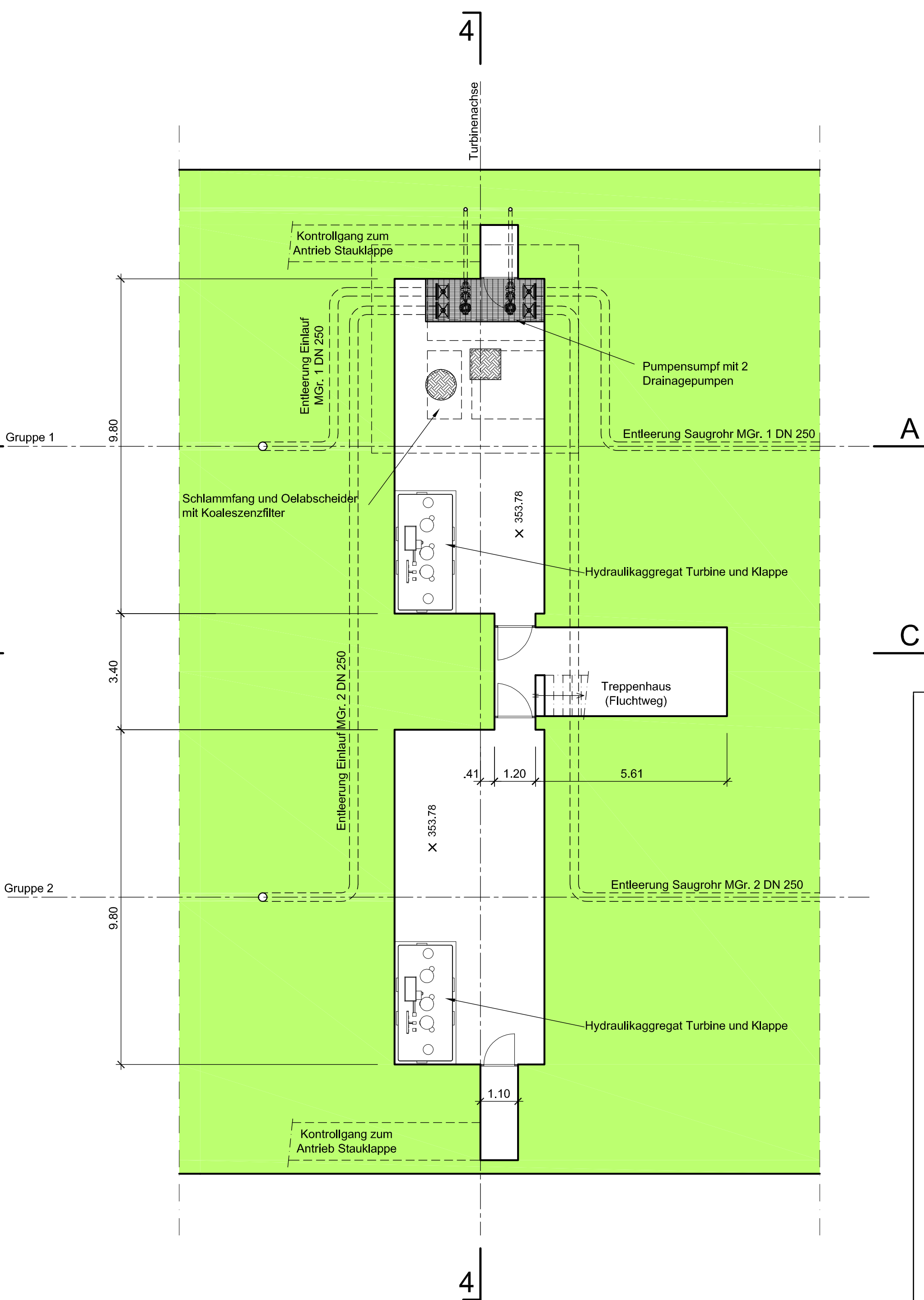
Grundriss auf Ebene Turbinengrube 1:100 Kote 353.78
