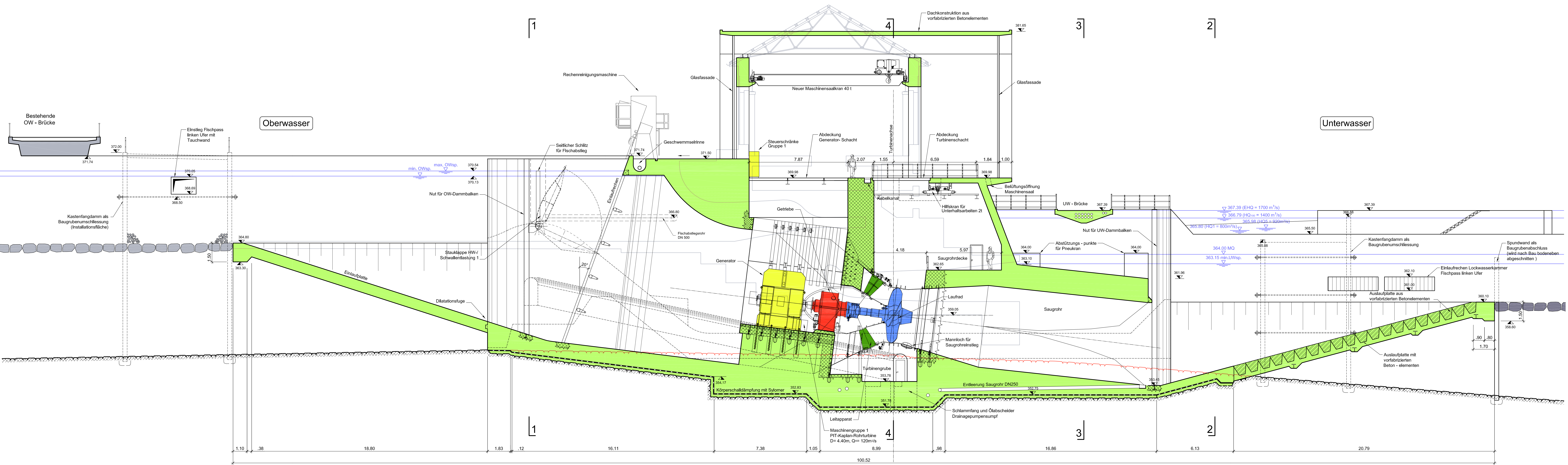
Längsschnitt A-A durch Maschinengruppe 1 1:100
