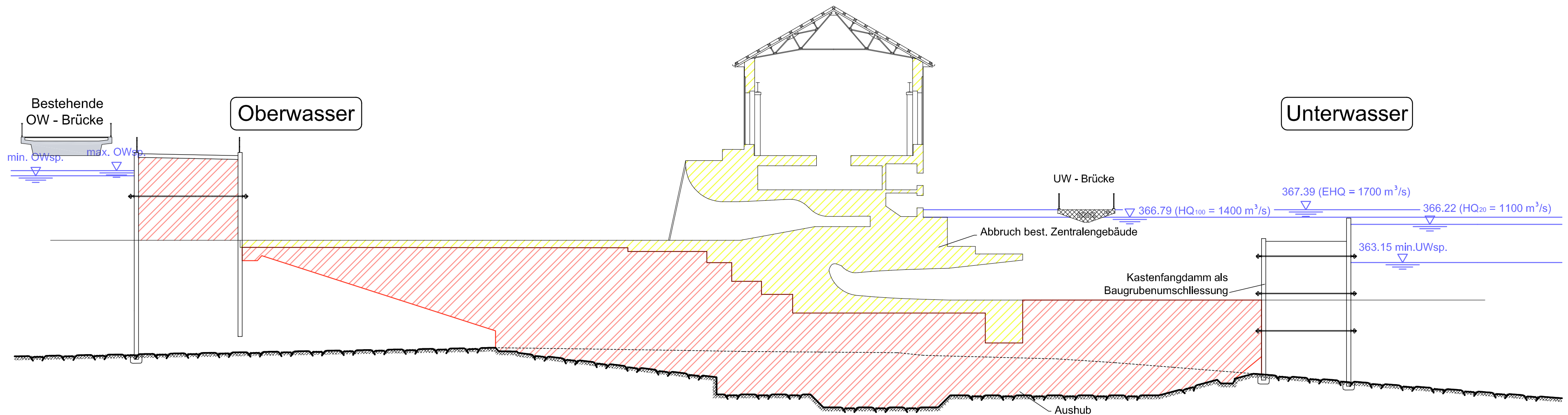
Längsschnitt durch Maschinengruppe 1:250
