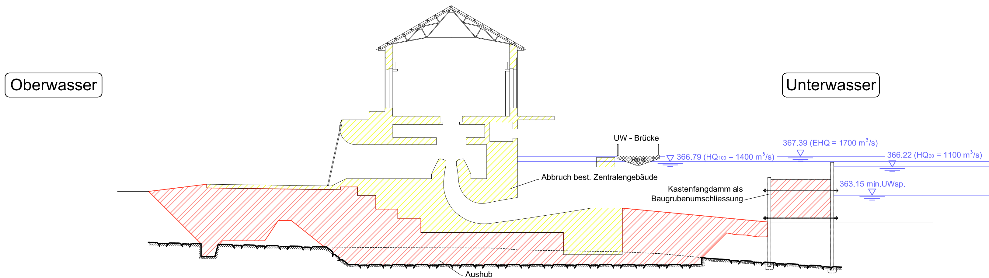
Längsschnitt durch Maschinengruppe 1:250
