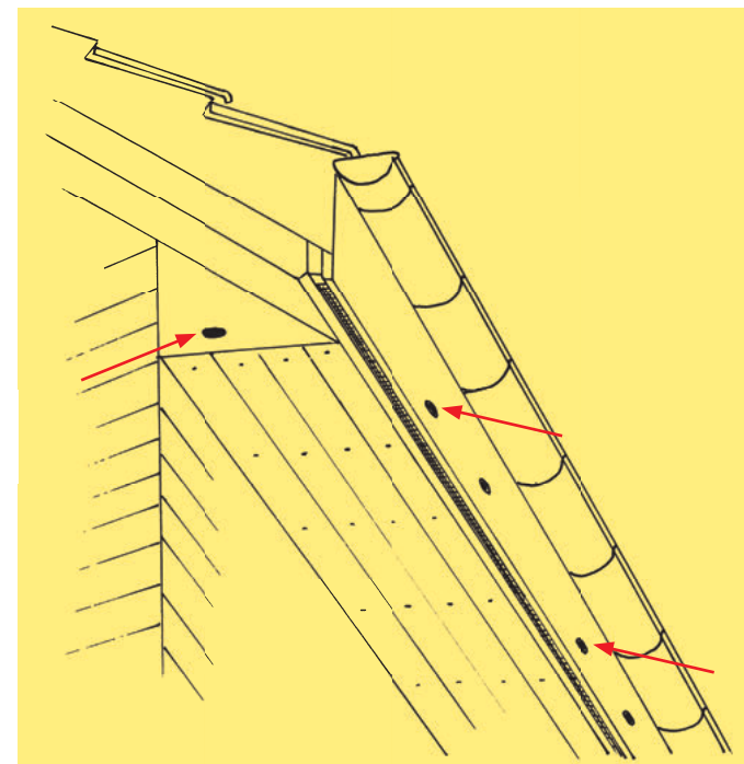
Nistplätze im Traufkasten. Die Abbildung zeigt Einflugöffnungen für Mauersegler unter der Regenrinne (im Stirnbrett) sowie eine Öffnung auf der Giebelseite.
