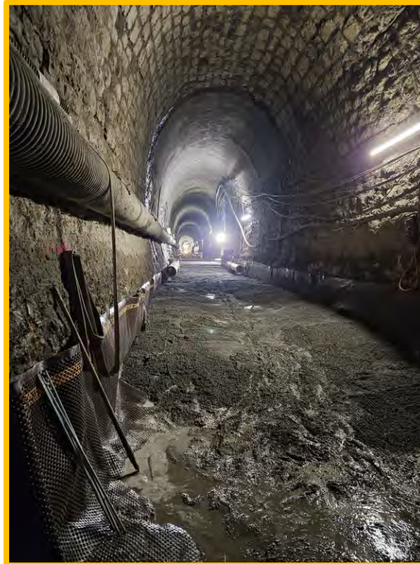
Betonarbeiten Sohle
