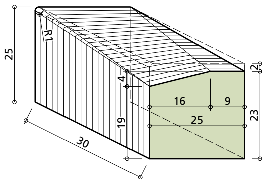
Absenkstein links Stellstein SN 25 vertikal / schräg
