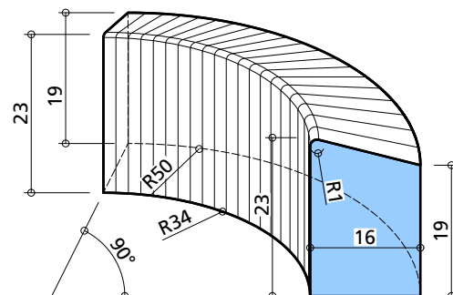
Insel-Eckstein Stellstein SN 16 schräg, Radius 50 cm
