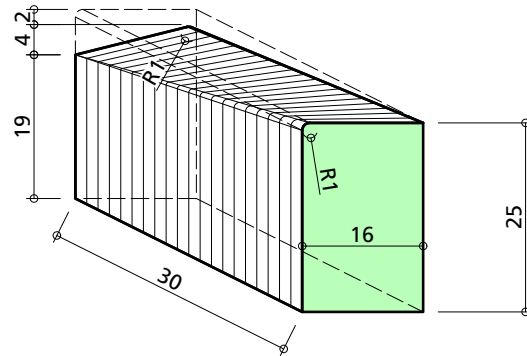
Absenkstein rechts Stellstein SN 16 vertikal / schräg
