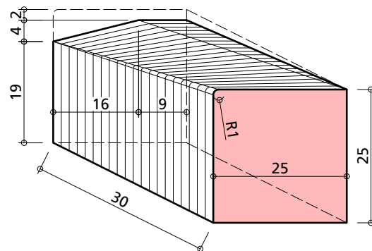
Absenkstein rechts Stellstein SN 25 vertikal / schräg
