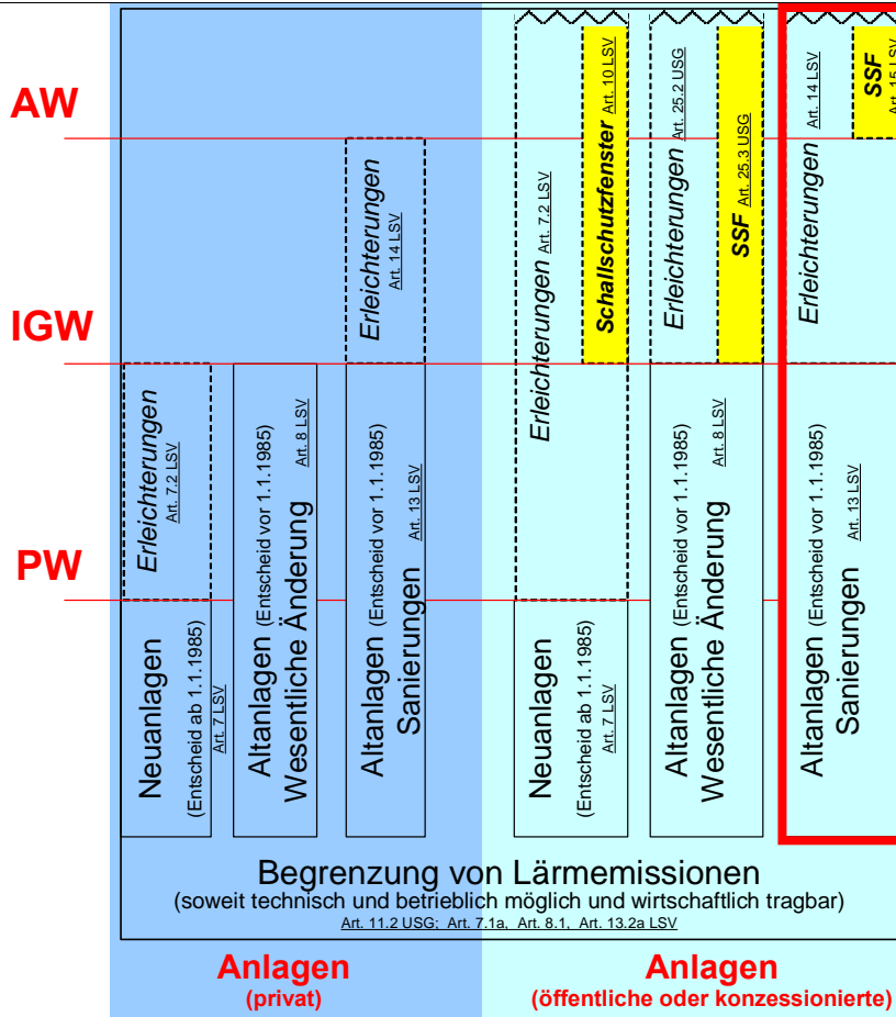
Abb. 1 > Geltungsbereich des Leitfadens (roter Kasten): Sanierung von öffentlichen Strassen.
