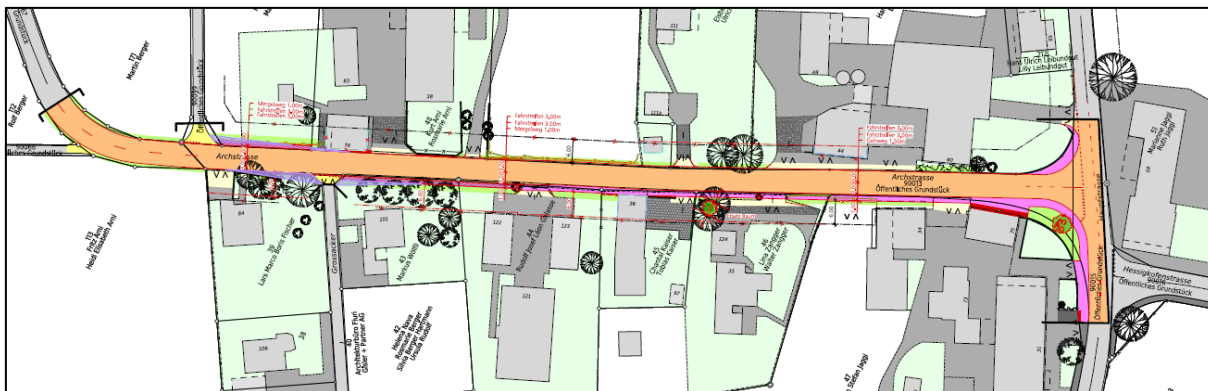
Abbildung 2, Übersicht Projektperimeter Strassen- und Werkleitungsbau
