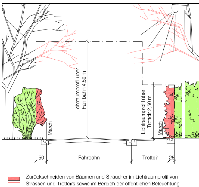
Abbildung 1, Lichtraumprofil Strasse
