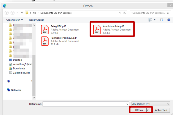
Abbildung 75 Explorer-Ansicht
