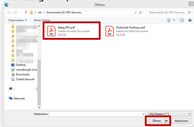
Abbildung 71 Explorer-Ansicht
