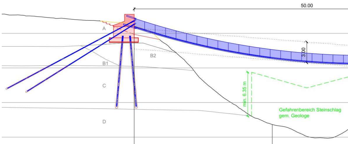
Abbildung 4: Längsschnitt der Brückenlösung, Teil West (Ausschnitt aus dem Übersichtsplan).
