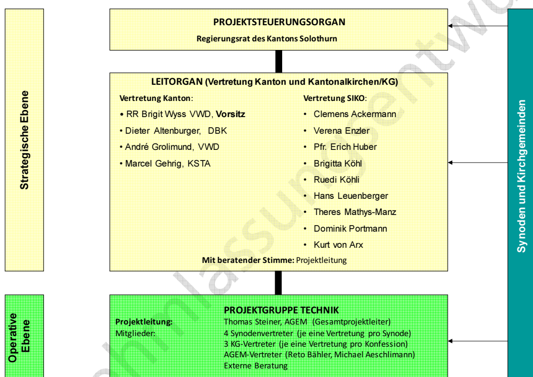
Abbildung 1-2: Projektorganisation
