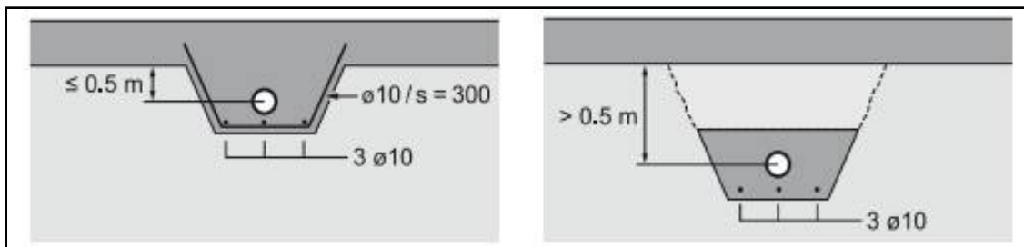
TWK 2017, S. 66 Kanalisationsleitung unter der Fundamentplatte
